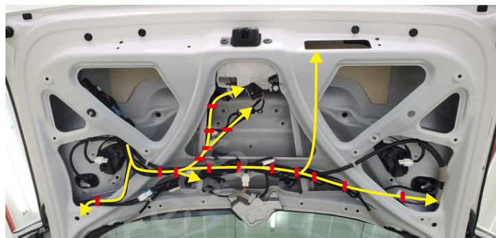
44. 用扎带沿着原车线束进行固定。
