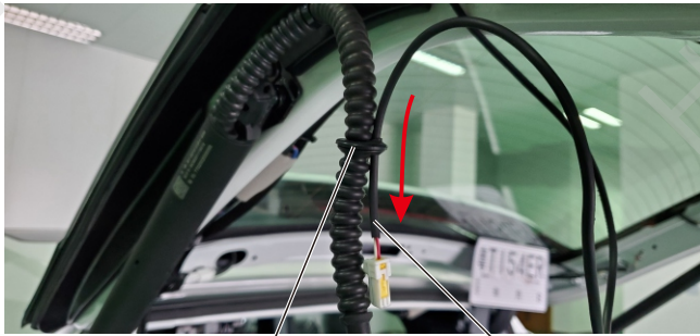
防水胶塞
