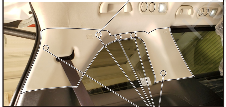
卡扣*5
